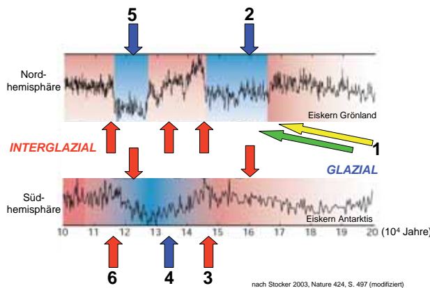
Schematische Darstellung der Funktionsweise der „bipolaren Klimamaschine“
